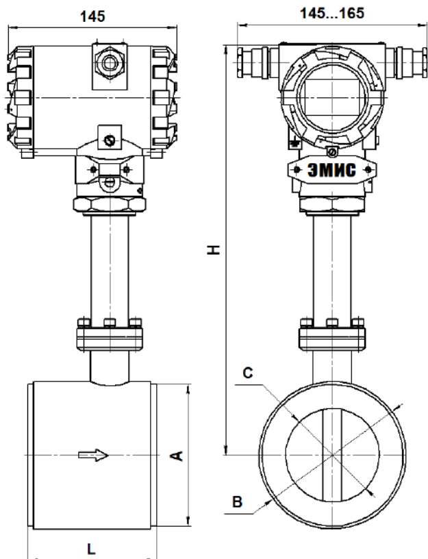
Рисунок В.2.1 (Ду15-100)
