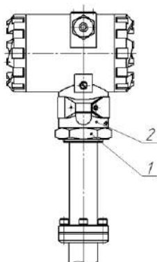
Рисуюнок 2.12 – Поворот электронного блока
