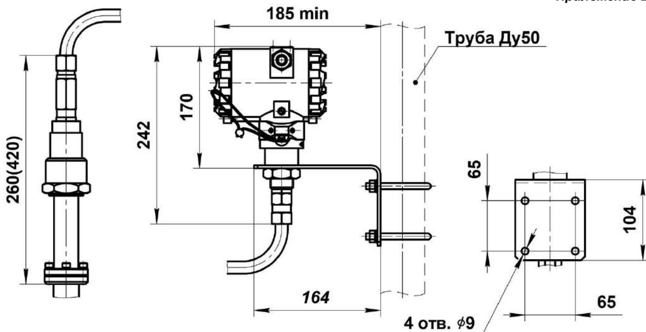
Рисунок В.11 - Размеры преобразователей дистанционного исполнения. Остальные размеры см. Рис.В.1 ...В.10
